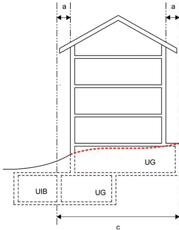
Fig. 6.2 Untergeschosse
