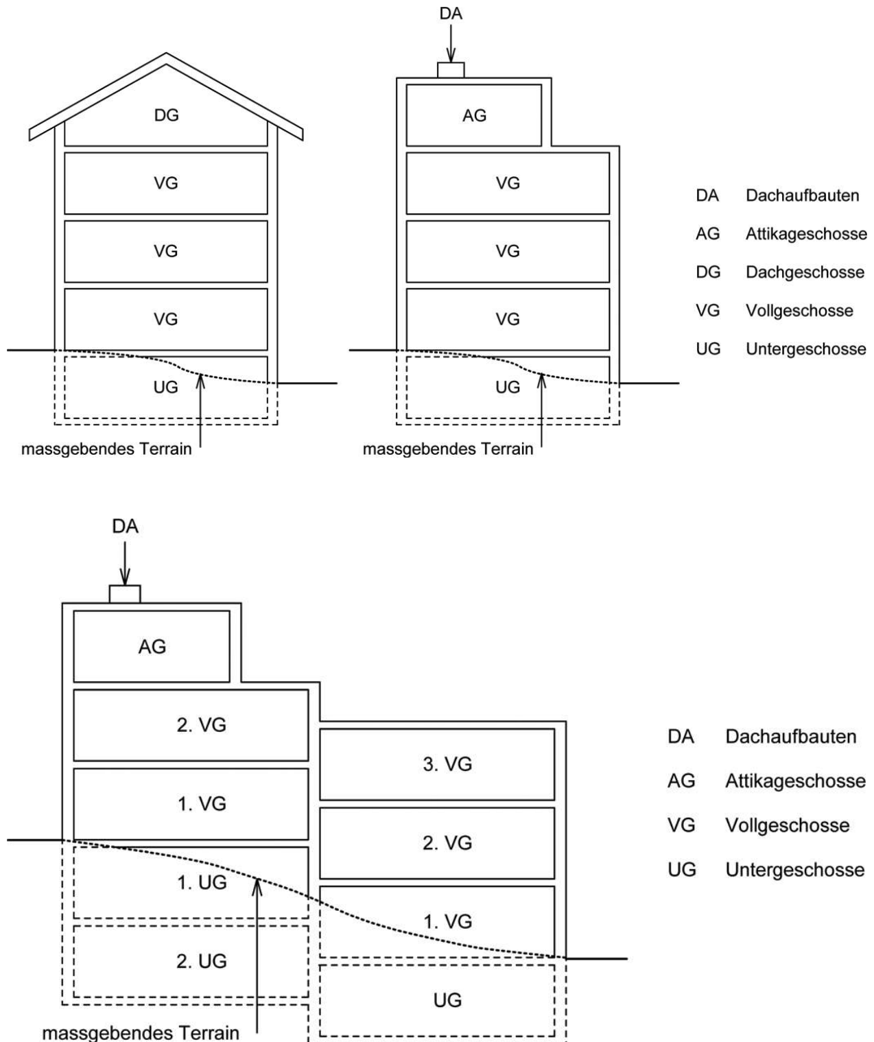
Fig. 6.1 Geschosse und Geschossezahl
