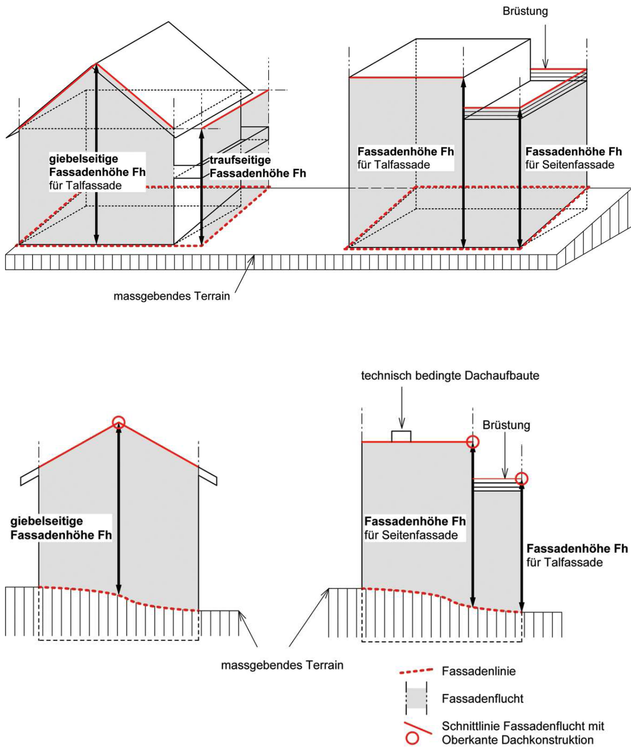
Fig. 5.2 Fassadenhöhe
