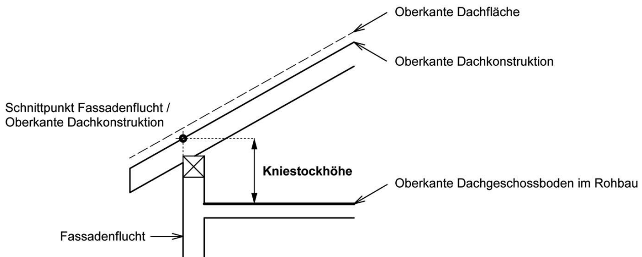
Fig. 5.3 Kniestockhöhe
