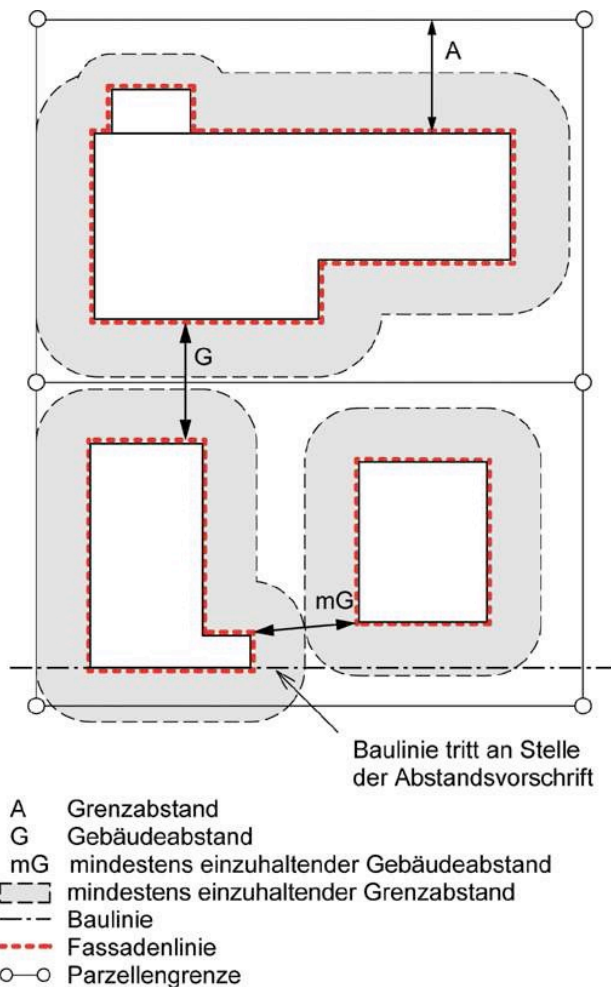
Fig. 7.1 - 7.3 Abstände und Abstandsbereiche
