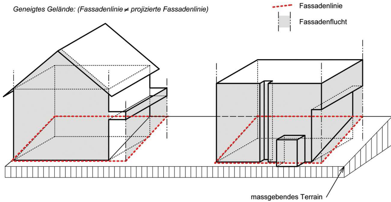
Fig. 3.1 – 3.2 Fassadenflucht und Fassadenlinie
