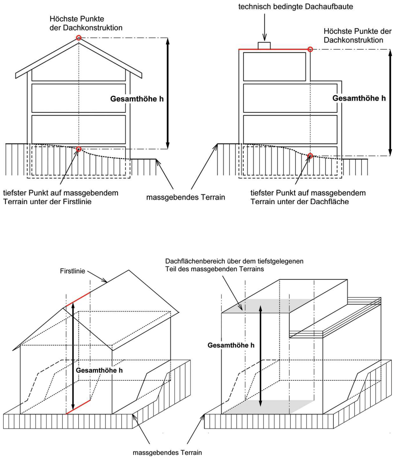
Fig. 5.1 Gesamthöhe
