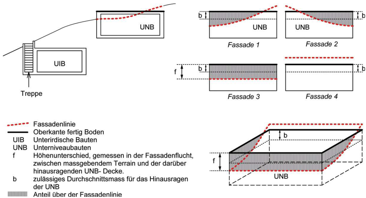
Fig. 2.4 – 2.5 Unterirdische Bauten, Unterniveaubauten
