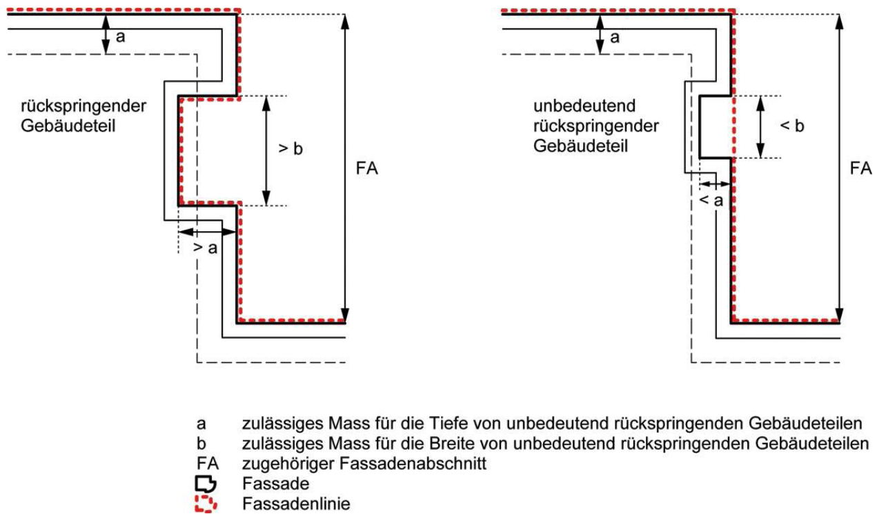
Fig. 3.5 Rückspringende und unbedeutende rückspringende Gebäudeteile
