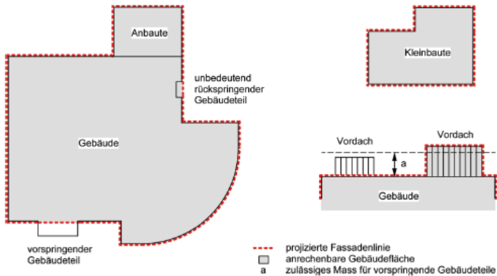
Fig. 8.4 Anrechenbare Gebäudefläche
