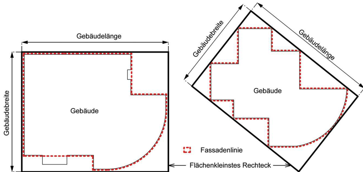
Fig. 4.1 und 4.2 Gebäudelänge und Gebäudebreite
