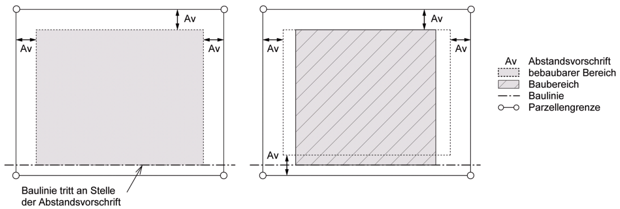
Fig. 7.4 Bebaubarer Bereich und Baubereich
