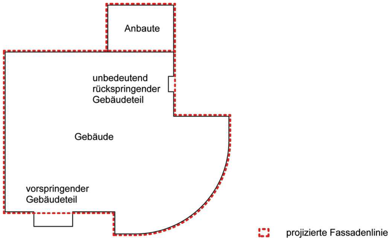
Fig. 3.1 – 3.2 Fassadenflucht und Fassadenlinie
