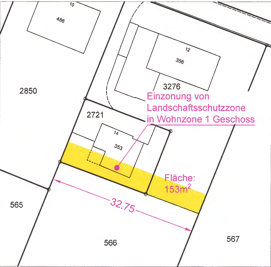
Ausschnitt aus amtlicher Vermessung 1:500
