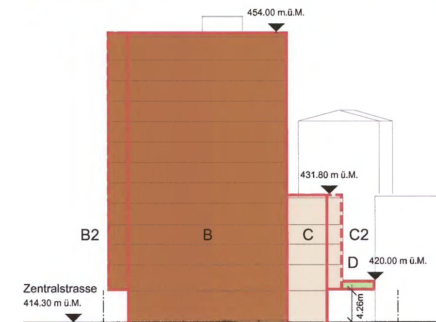
Nordostfassade b-b
