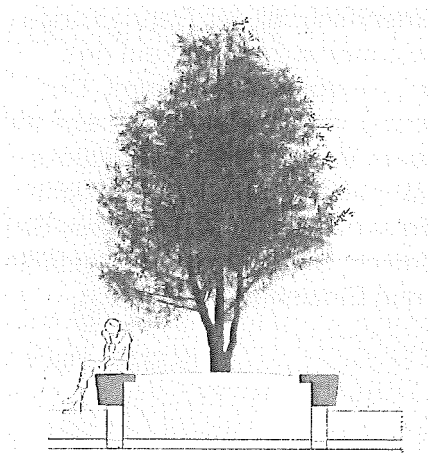
Schemaschnitt Pflanztrog mit Gehölz
