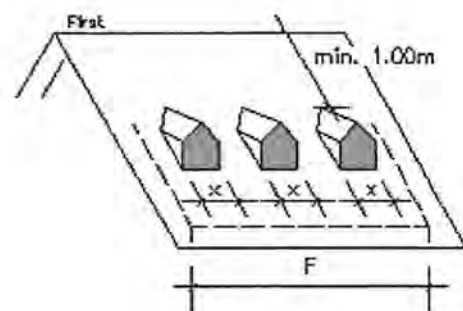
Giebelgauben (Lukarnen)
