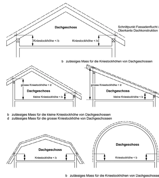
Abbildung 10: Dachgeschosse (Ziff. 6.3 Anhang zum Baugesetz)
