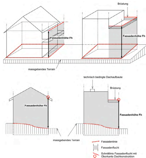
Abbildung 7: Fassadenhöhe (Ziff. 5.2 Anhang Baugesetz)
