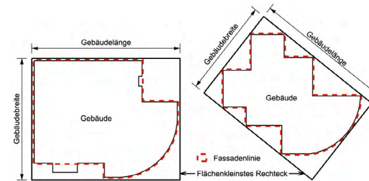
Abbildung 5: Gebäudelänge (Ziff. 4.1 Anhang Baugesetz)
