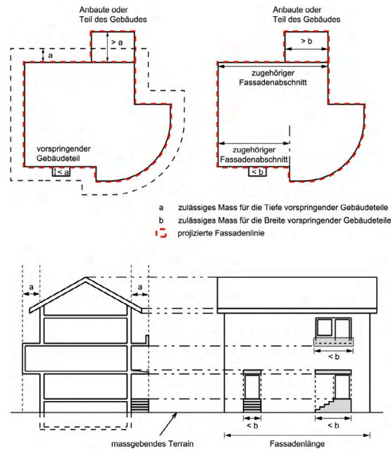
Abbildung 4: Vorspringende Gebäudeteile (Ziff. 3.4 Anhang Baugesetz)
