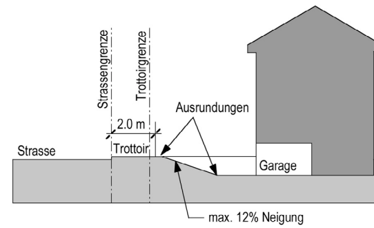
Abbildung 14: Garagenhofzufahrt, Garagenvorplatz (Art. 43 Abs. 1)
