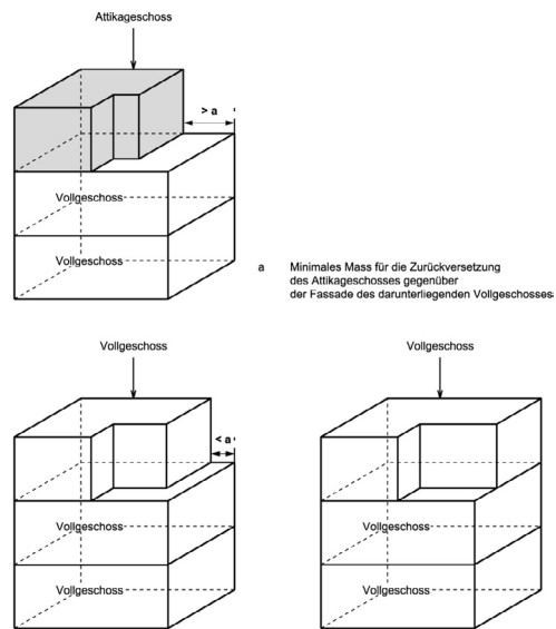
Abbildung 11: Attikageschosse (Ziff. 6.4 Anhang zum Baugesetz)
