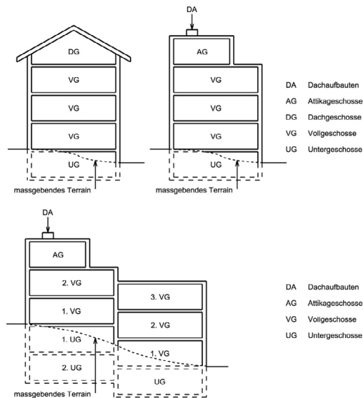
Abbildung 8: Vollgeschosse (Ziff. 6.1 Anhang Baugesetz)
