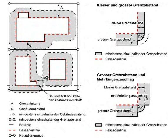
Abbildung 1: Grenz- und Gebäudeabstand (Ziff. 7.1 und 7.2 Baugesetz)
