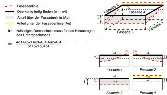
Abbildung 3: Unterirdische Bauten, Unterniveaubauten (Ziff. 2.4 und 2.5 Anhang Baugesetz, Skizze ergänzt)
