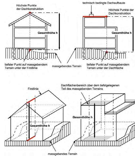
Abbildung 6: Gesamthöhe (Ziff. 5.1 Anhang Baugesetz)
